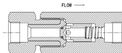
中压软密封单向阀
